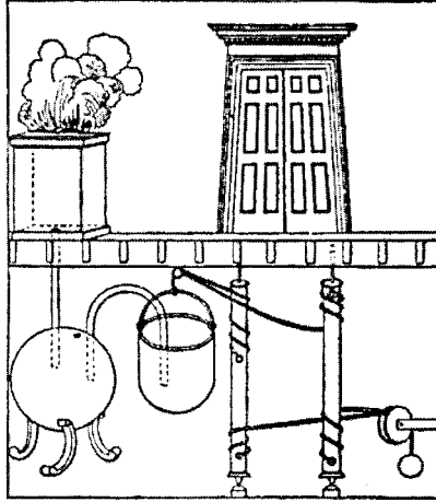
من مخترعات هيرو: الشكل الأعلى: أبواب معبدٍ تُفَتِّحُ بنايِرٌ تُوقَدُ على مذابح القرابين. الشكل الأسفل: محرِّك بخاري.
